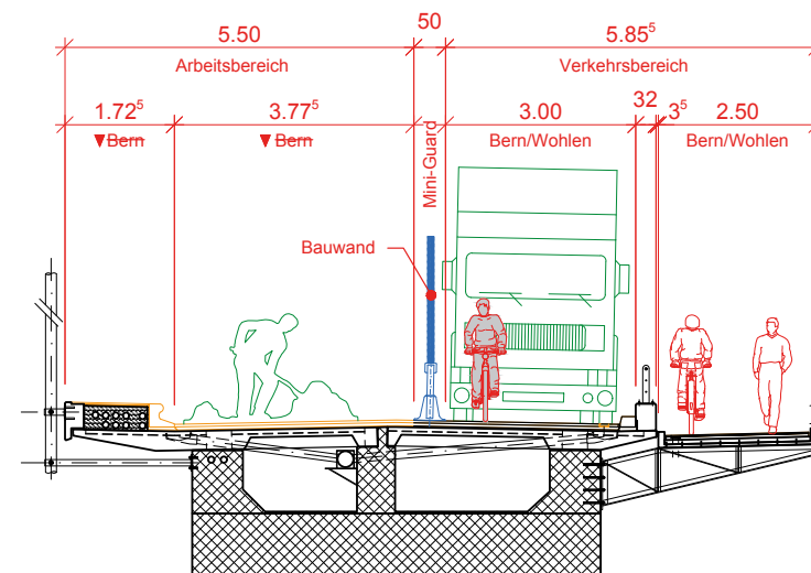
Querschnitt, Zweite Bauphase
