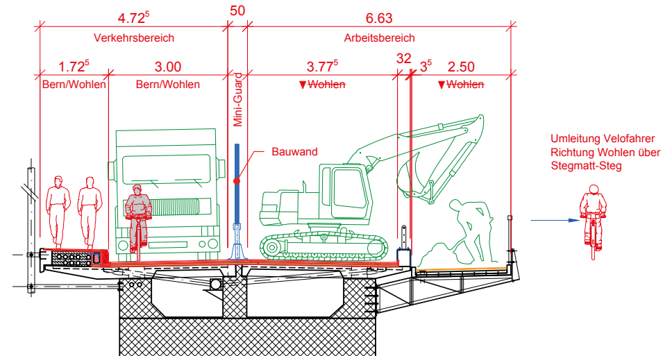
Querschnitt, Erste Bauphase
